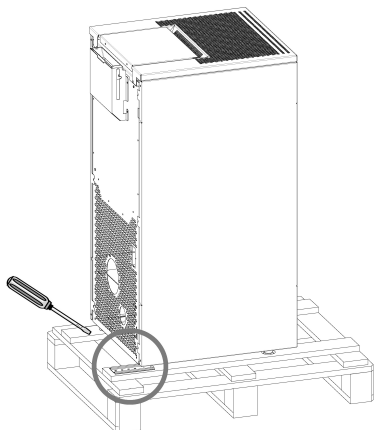
Fig. 1 - Verwijdering van de beugels
