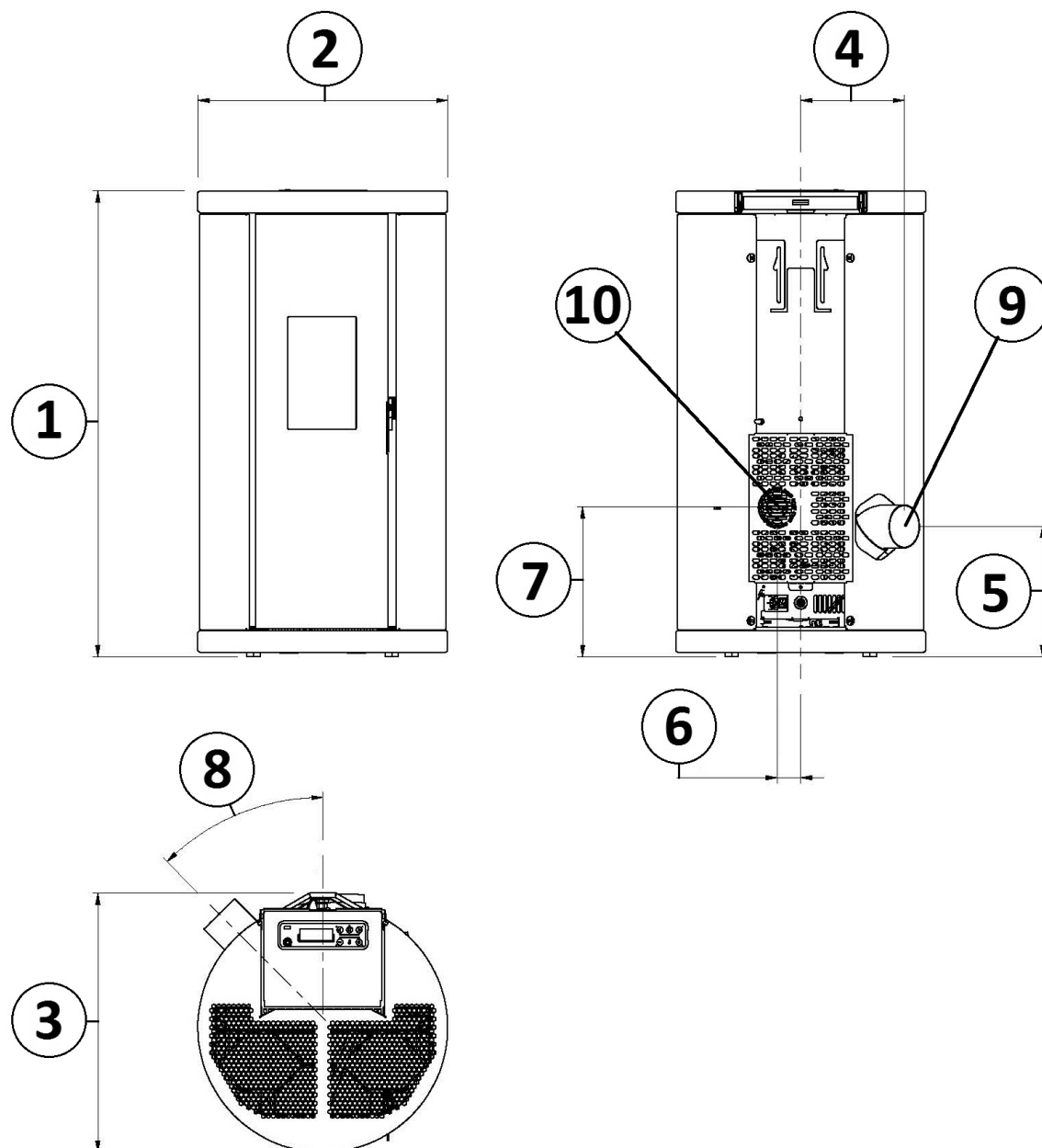
Fig. 15 - Algemene afmetingen: Rondò 3
