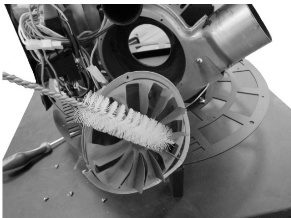
Fig. 45 - Reiniging rookgassenafzuiger: fase 1
