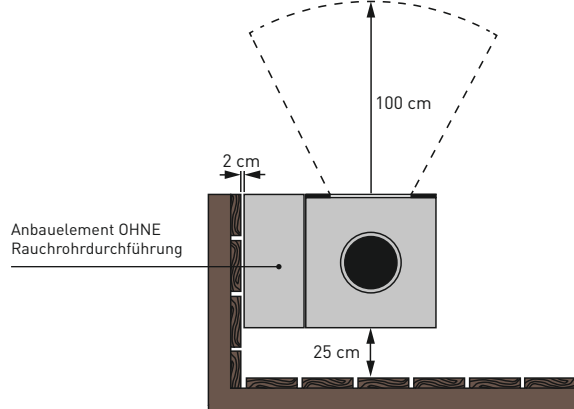
Draufsicht Brennkammer
