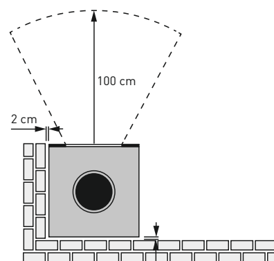
Draufsicht Brennkammer
