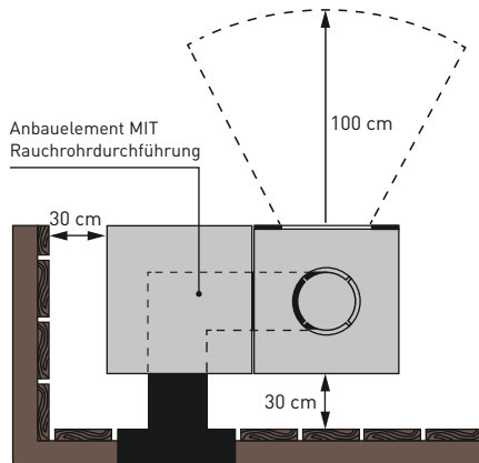
Draufsicht Brennkammer
