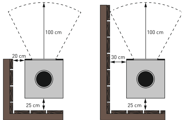
Draufsicht Brennkammer
